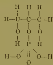
C_3H_9PO_6 Glycerinphosphorsäure.
